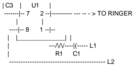
a. Main ringer TTL circuit
